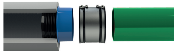
Verbinding naar tapse aansluiting d.m.v. een standaard SC koppeling, met of zonder reduceerring...
