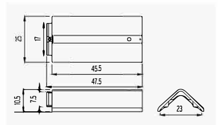
6 Hoekige vorst 100°
