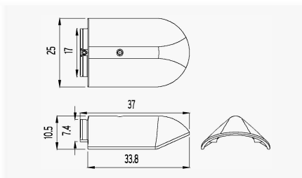
7 Hoekige beginnoordboom 100°
