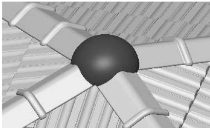
7 Hoekige beginnoordboom 100°
