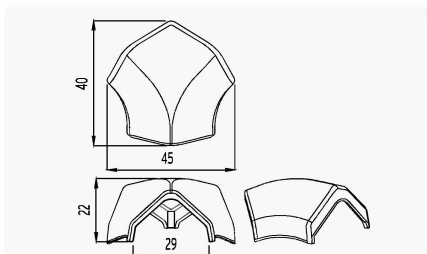
8 Verbindingsstuk 3 richtingen 100°
