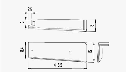
11 Linkse gevelpan FLAT-5XL®
