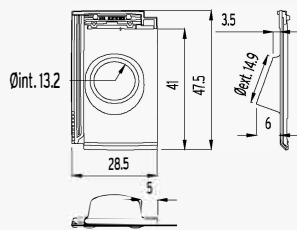
22 Haard doorvoerpan FLAT-10
