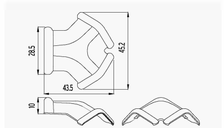
3 Verbindingsstuk 3 richtingen
