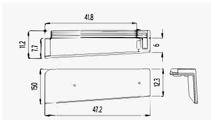
13 Rechtse gevelpan
