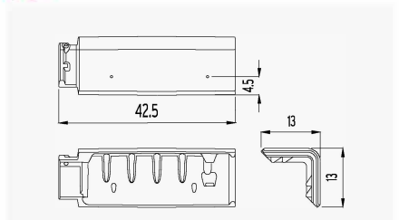
15 Universele gevelpan (EENZIJDIGE VORSTAANSLUITING)
