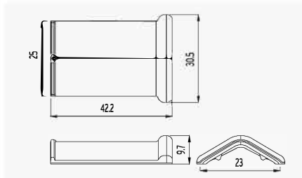
1 Hoekige vorst
