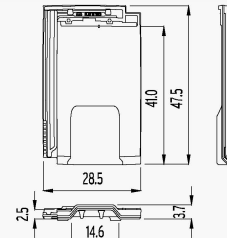
24 Ventilatiepan FLAT-10
