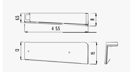
12 Linkse gevelpan
