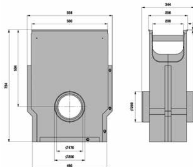
Zandvanger met verzinkt stalen emmer
