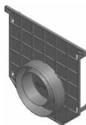
Sluitstuk type 01, in PE-PP, met uitloop DN 75/110
