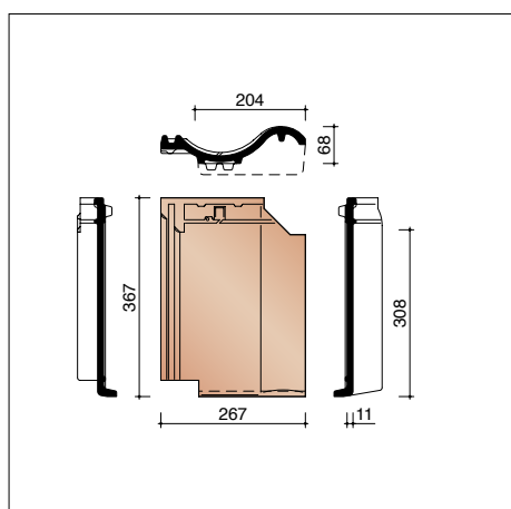
JOVH8300 4,9 pièces/m crt Tuile à bord recourbé
