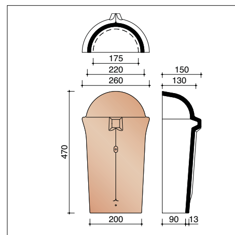
J/N0003110 About d'arêtier conique
