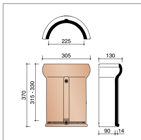
J/N0001200 3 - 3,1 pièces/m crt Faîtière/arêtier demi-rond(e) Vario - 225 mm
