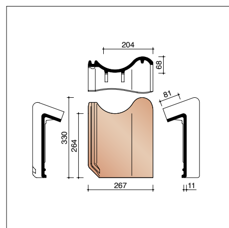
JOVH8500 4,9 pièces/m crt Tuile faîtière
