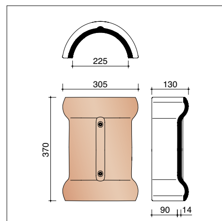
J/N0001250 Faîtière demi-ronde Vario à double bourrelet - 225 mm
