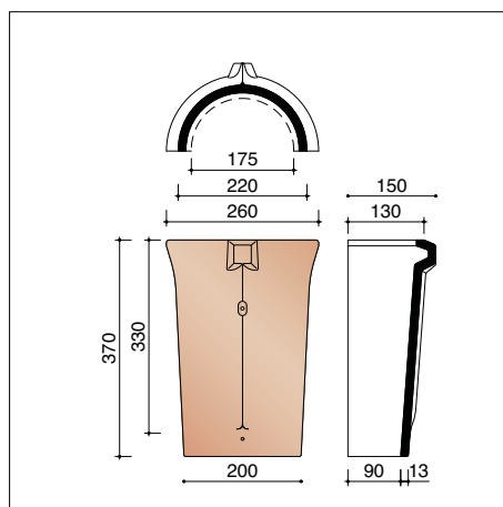
J/N0003100 3 pièces/m crt Arêtier conique
