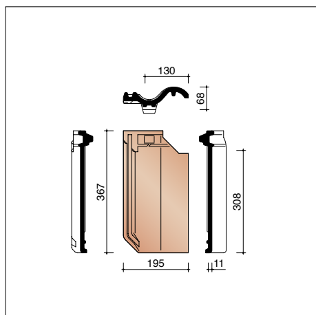
JOVH8010 3,2 pièces/m crt Demi-tuile
