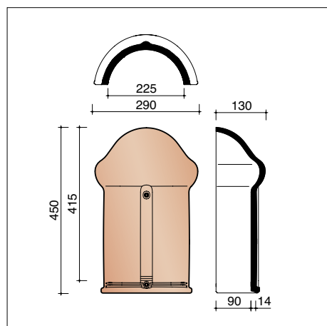
J/N0001260 About d'arêtier demi-rond Vario - 225 mm
