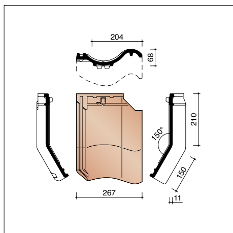
JOVH8200 4,9 pièces/m crt Tuile membron 150°
