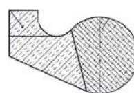
Verrouillage par verrous et cordon de soudure
