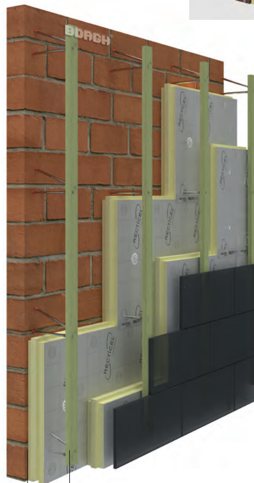
Facafix XL Encorbellement 210 - 320
