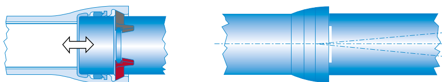
Verrouiller l'assemblage
